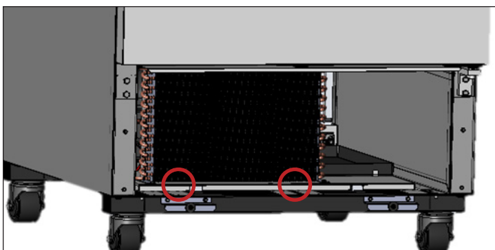
Rys. 5. Odkręcić śruby u podstawy skraplacza.
