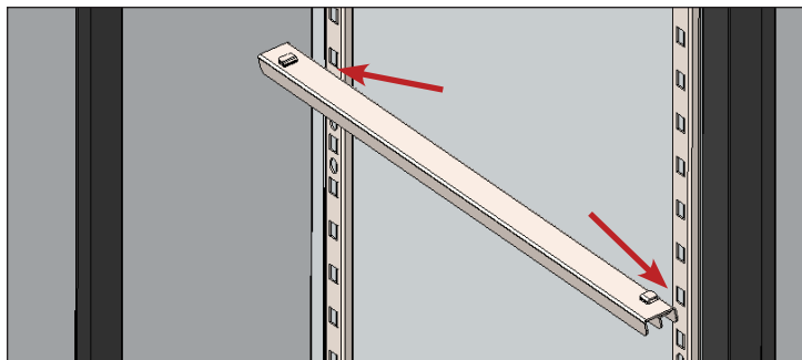
Rys. 1. Ustawić wypustki naprzeciwko otworów.
