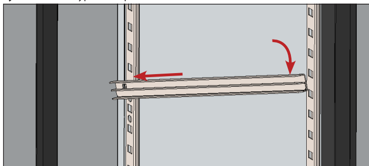
Rys. 2. Włożyć prowadnicę półki/tacy.
