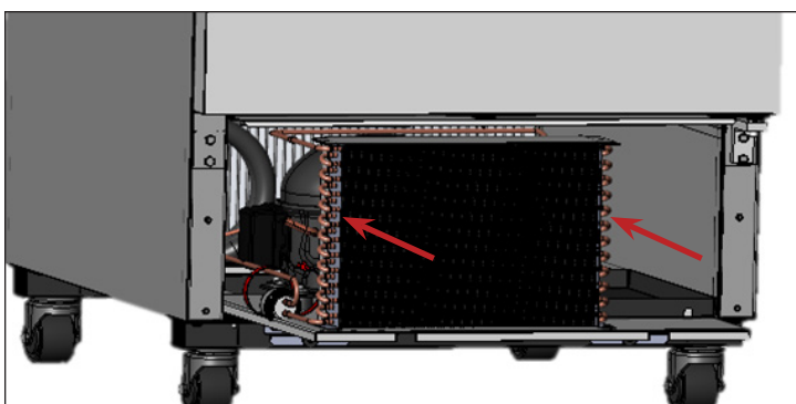
Rys. 7. Ostrożnie z powrotem wsunąć zespół skraplacza na swoje miejsce i wkręcić śruby.
